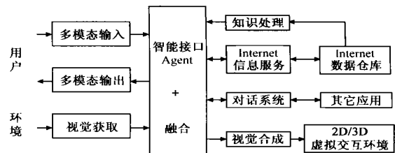
图 1 第四代人机交互通讯概念模型
