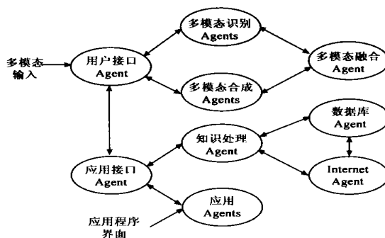
图 2 第四代人机自然交互与通信多 Agent 结构模型
