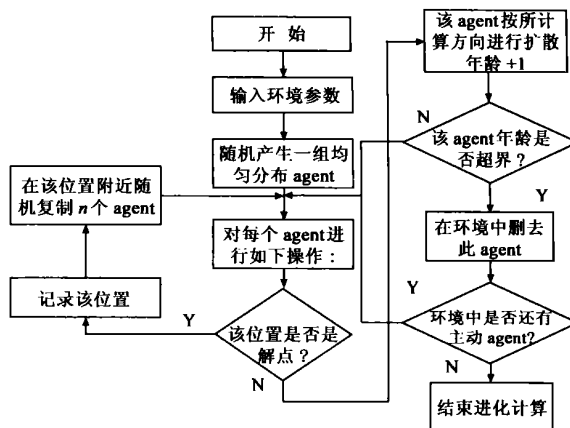
图 7 进化 Agent 的计算流程
