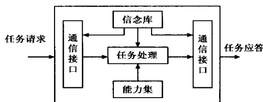
图 4 人机交互 Agent 的基本模型
