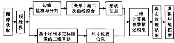
图 14 AVR 重建算法的基本流程
