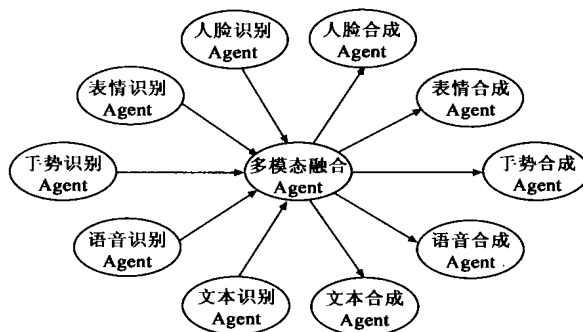
图 3 多模态感知部分 Agent 结构模型
