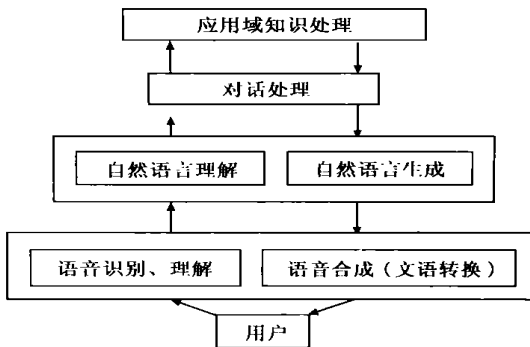
图 11 人机自然交互过程的分层结构
